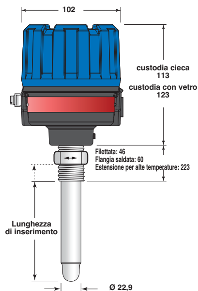
Modello TD2 con elettronica integrata e sensore ad estremità sferica TMA/TMB
