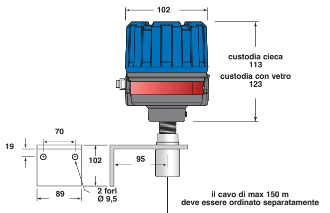
Modello TD2 con elettronica remota
