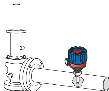
Monitoraggio valvole di sicurezza
